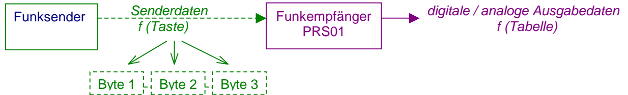
Informationsfluss
