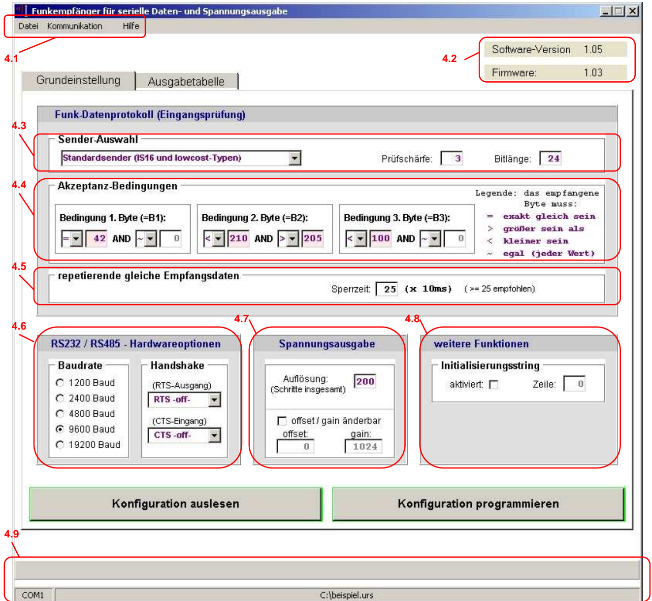
Konfigurationssoftware: Grundeinstellung
