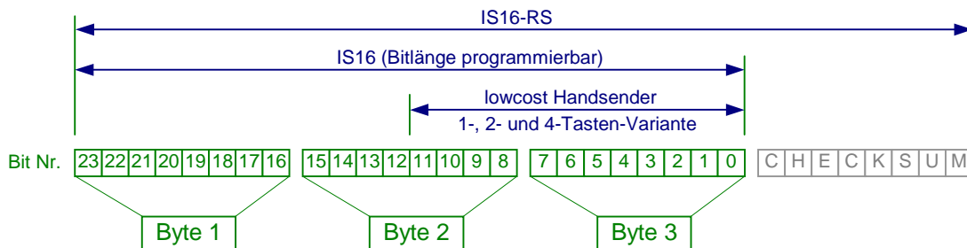
Aufbau Senderdaten
