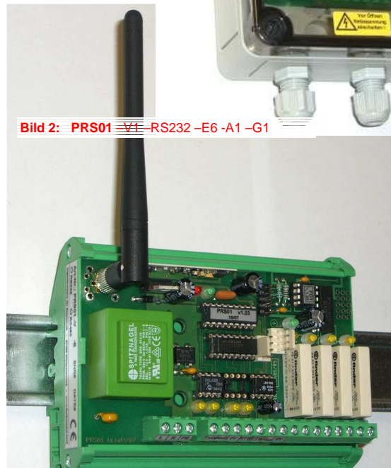
Bild 3: PRS01 mit Erweiterung 4xRelais Schliesser 5A/250VAC
